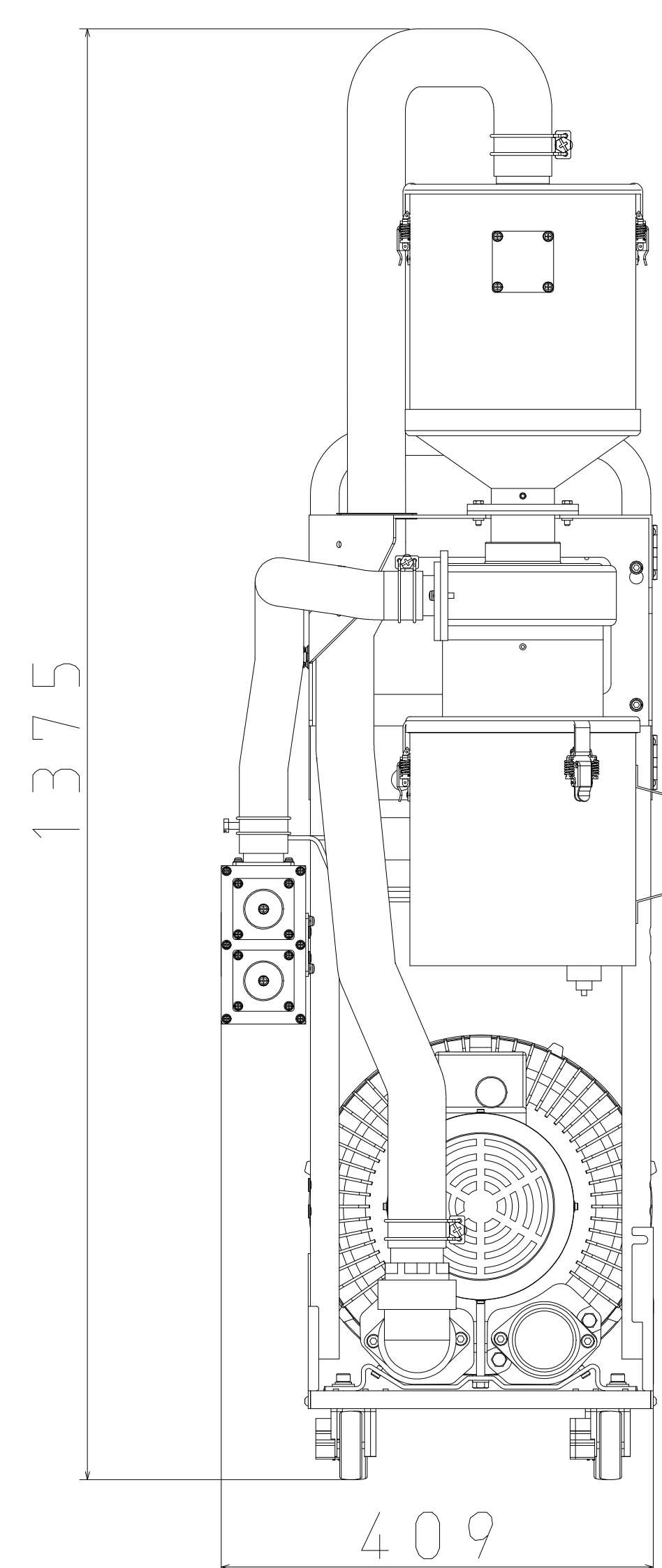
TL 集塵サイクロン付
