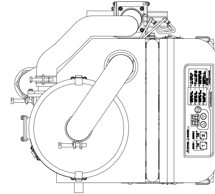
TL 集塵サイクロン付
